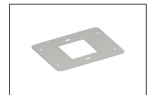
KT230/IS Placa de fijacion en acero inoxidable AISI 304, equipada con tirantes y tornillos para BI/001PE - BI/001PC - BI/004HP - BI/006.
