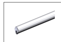
BA/90/6 Mástil de aluminio pintado de blanco, longitud de 6 metros, con perfil de cubierta LED y caucho goma antichoque.
